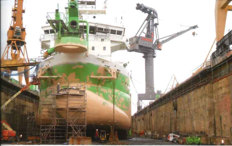
DRY DOCK N° 2 (230X33 M) CRANES: 200 / 40 / 15 T. 2 PITS
