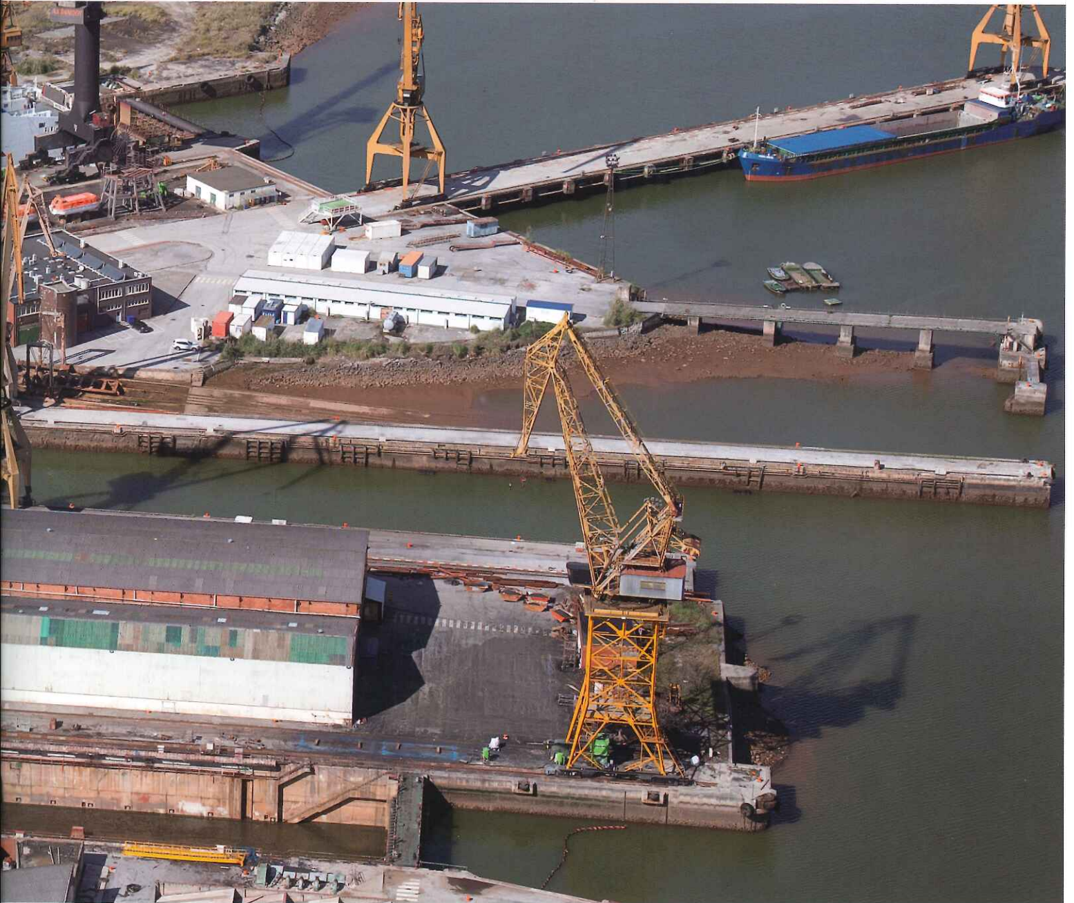
DRY DOCK N° 2 (230X33 M) CRANES: 200 / 40 / 15 T. 2 PITS
